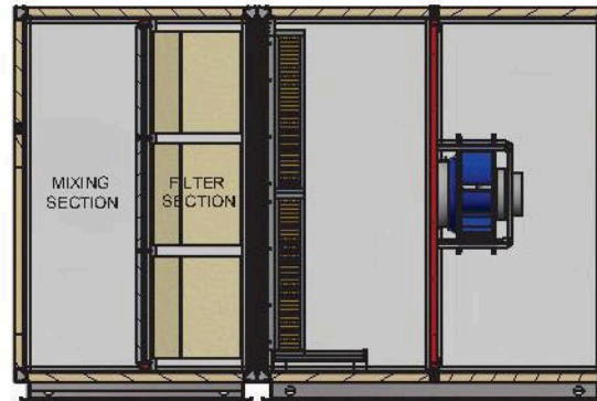
A-A (1 : 32)
